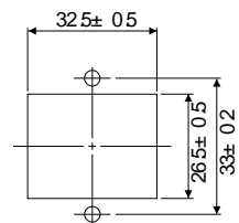
パネルカット寸法
