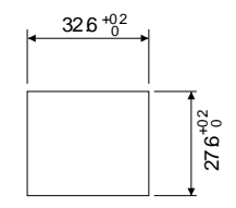
パネルカット寸法
