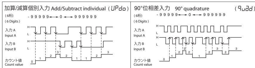
オープンコレクタ入力の例 The example shown is open collector input mode.
