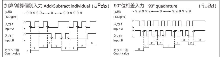
オープンコレクタ入力の例 The example shown is open collector input mode.
