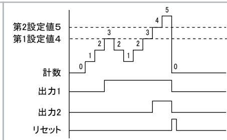
2段設定、オーバーラン式自己保持出力
