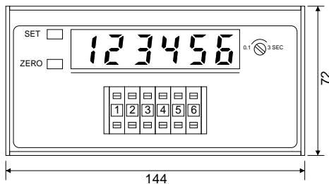
MDR-266M
